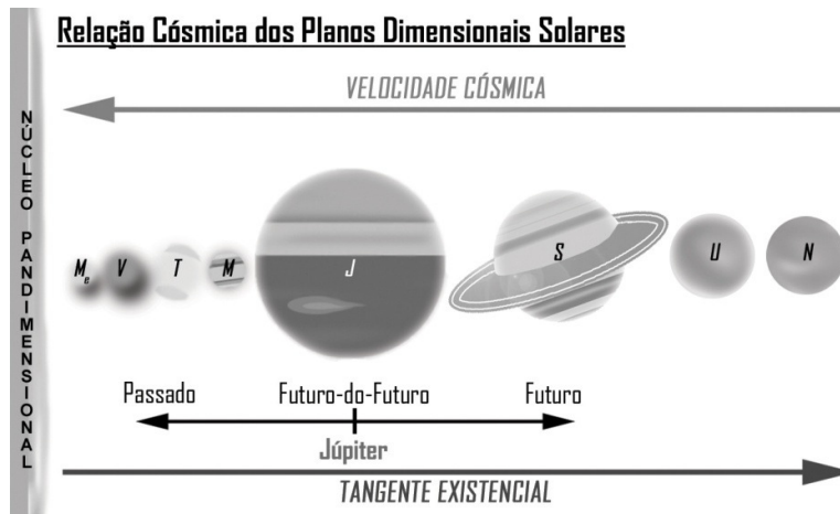
Da esquerda para direita, os planetas: Mercúrio, Vênus, Terra, Marte, Júpiter, Saturno, Urano e Netuno; planetas que formam o bloco G8 .
